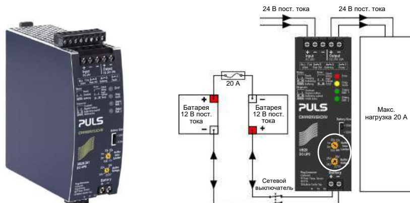
Рисунок 28. Конфигурация DC-UPS и батарей
