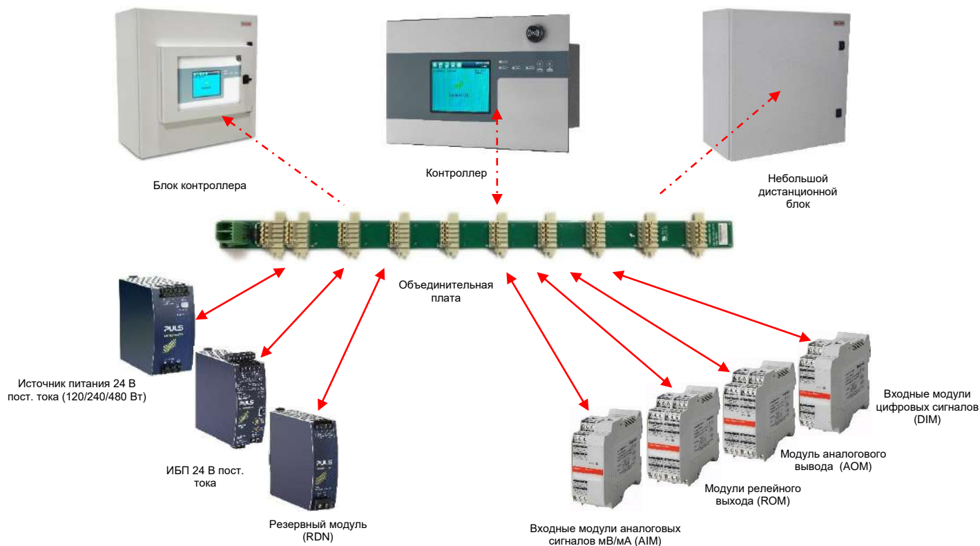
Рисунок 16. Структурные элементы системы TPPR
