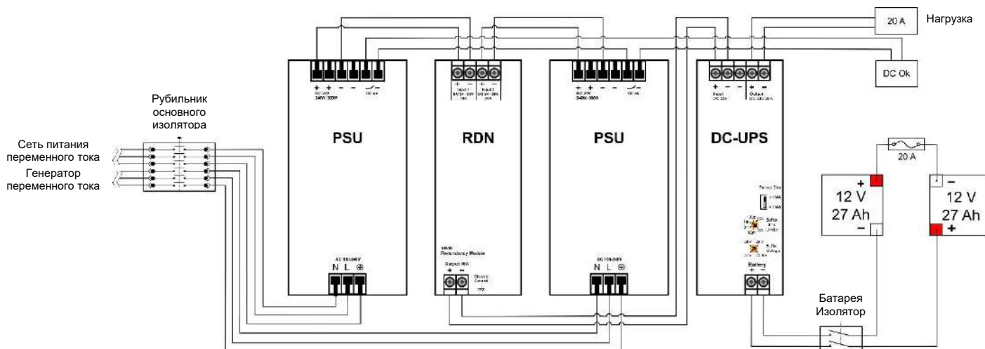
Рисунок 25. Типичная схема подачи питания
