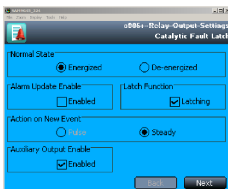
Рисунок 38. Конфигурация фиксации выхода при неисправности
