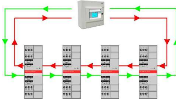
Рисунок 23. Пример кольцевого контура
