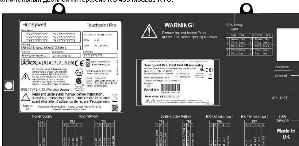
Рисунок 19. Крышка контроллера TPPR с картой соединений
