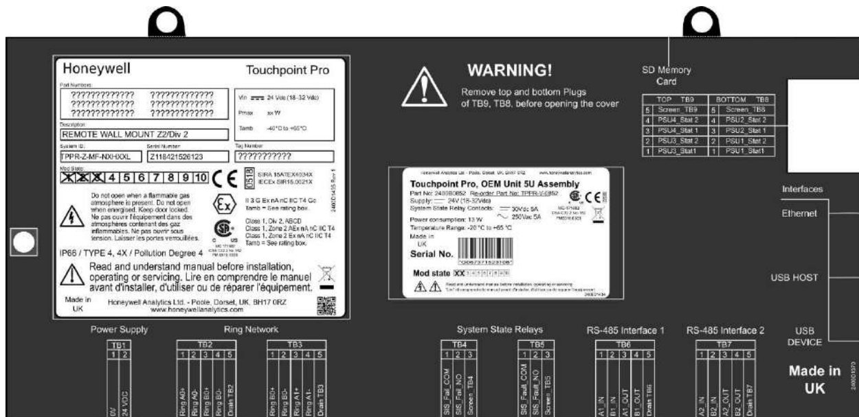
Рисунок 5. Задняя крышка контроллера с примерами ярлыков
