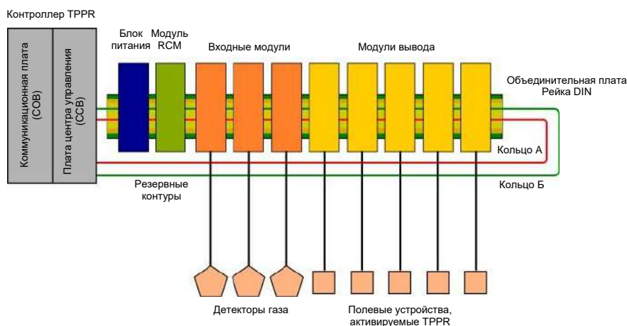
Рисунок 22. Схема типичного контроллера TPPR
