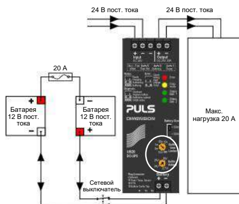
Рисунок 29. Цепь батареи
