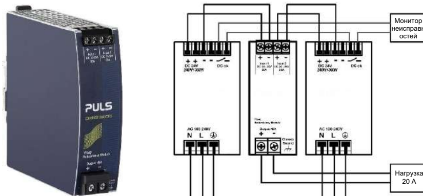
Рисунок 27. Эксплуатация резервного модуля питания
