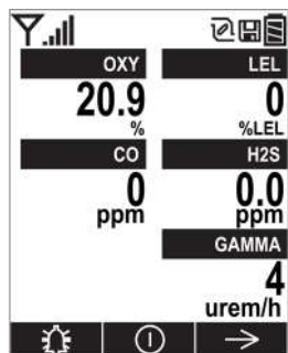
Пять датчиков, в том числе датчик гамма-излучения.
